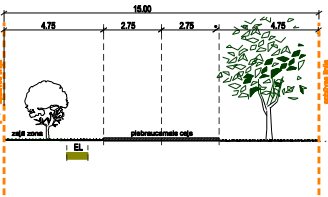
Iekškvartāla ceļš 15m GRIEZUMS I - I
