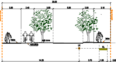
Iekškvartāla ceļš 20m GRIEZUMS K-K
