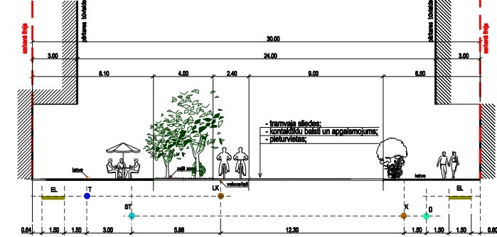
GĀJĒJU PROMENĀDE sarkanās līnijas 30m GRIEZUMS A - A
