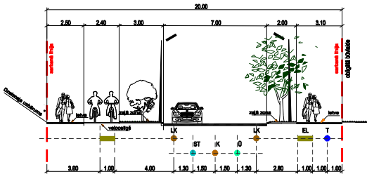
Jaunā iela sarkanās līnijas 20m GRIEZUMS C2-C2
