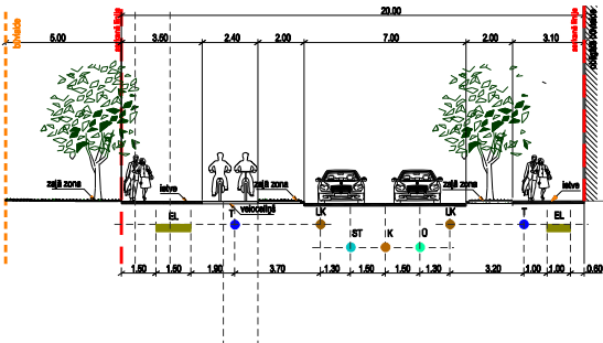
Jaunā iela sarkanās līnijas 20m GRIEZUMS C1-C1
