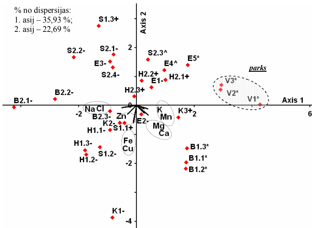
4.18. att. Pētīto parauglaukumu liepu lapu ķīmiskā sastāva (2005. g. augusta dati) izvietojums ar komponentanalīzi nodalītājās asīs. (* - veselīga; ^ - viegli bojāta; + - vidēji bojāta un – stipri bojāta liepa).
