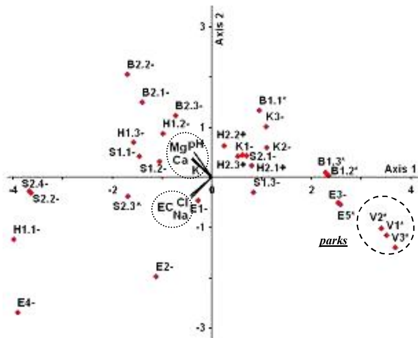
4.4. att. Pētīto parauglaukumu sniega ūdens ķīmiskā sastāva (2004. gada 26. novembra dati) izvietojums ar komponentanalīzi nodalītajās asīs. (* - veselīga; ^ - viegli bojāta; + - vidēji bojāta un - stipri bojāta liepa.)
