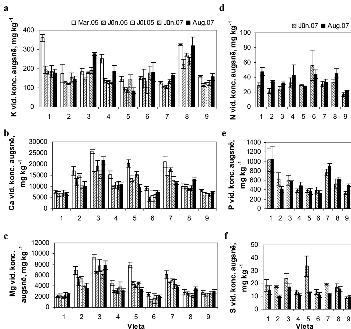
3.16. att. Makroelementu koncentrācija ( \text{mg} \cdot \text{kg}^{-1} ) Rīgas ielu apstādījumu augsnē 2005. un 2007. gadā (vidējā koncentrācija 3-5 pētījuma vietas kociem \pm \text{SE} ).
