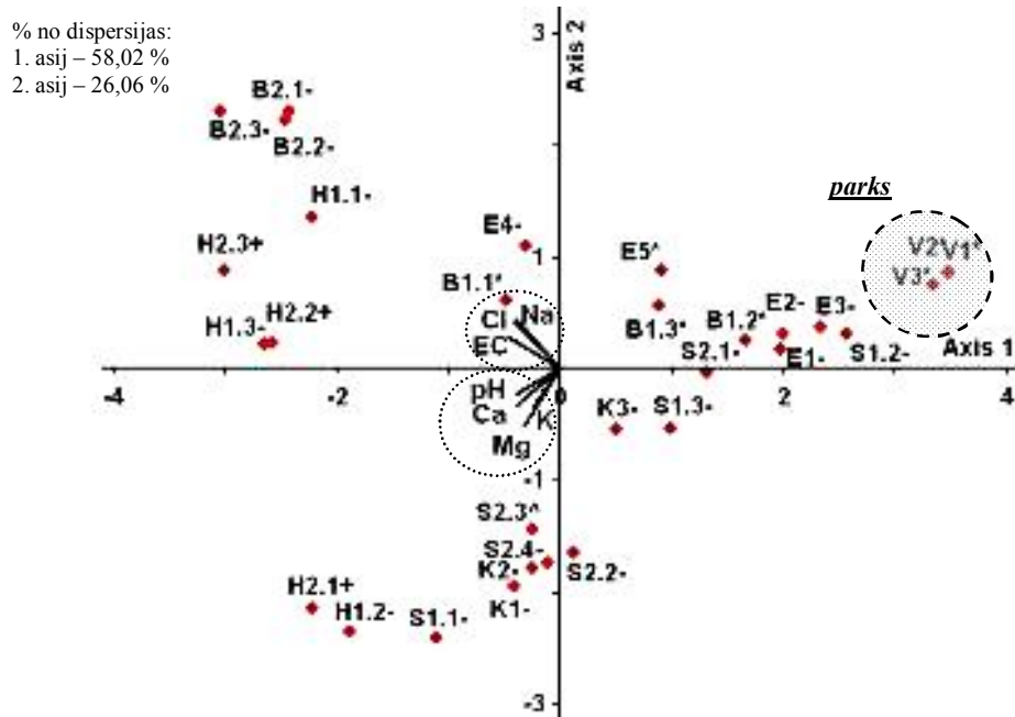
4.6. att. Pētīto parauglaukumu sniega ūdens ķīmiskā sastāva (2004. gada 28. decembra dati) izvietojums ar komponentanalīzi nodalītajās asīs. (* - veselīga; ^ - viegli bojāta; + - vidēji bojāta un – stipri bojāta liepa.)
