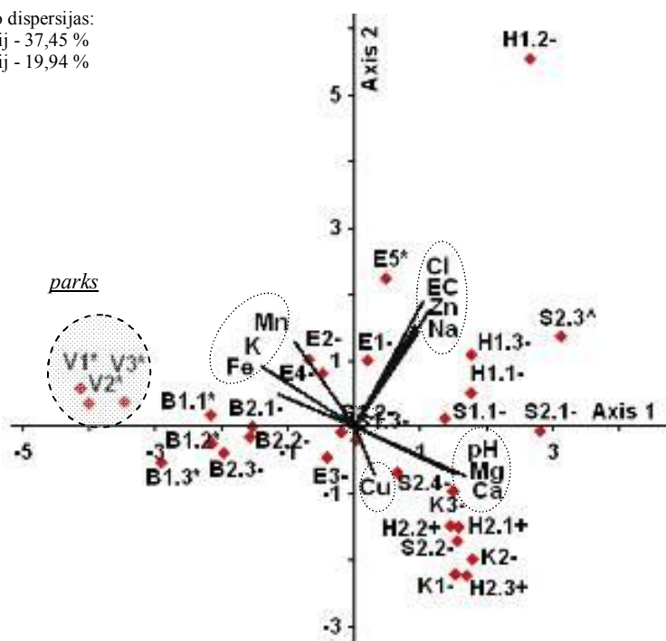
4.9. att. Pētīto parauglaukumu augšņu ķīmiskā sastāva (2005. gada marta dati) izvietojums ar komponentanalīzi nodalītājās asīs. (* - veselīga; ^ - viegli bojāta; + - vidēji bojāta un – stipri bojāta liepa.)
