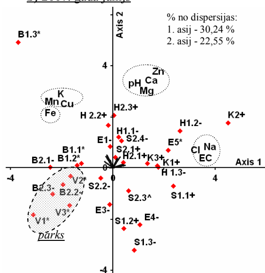
4.10. att. Pētīto parauglaukumu augšņu ķīmiskā sastāva (2005. (a) un 2007. gada (b) jūnija dati) izvietojums ar komponentanalīzi nodalītājās asīs. (* - veselīga; ^ - viegli bojāta; + - vidēji bojāta un - stipri bojāta liepa.)
