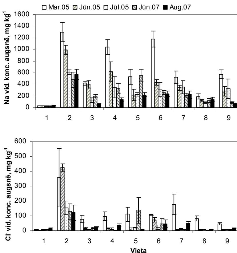
3.15. att. Na un Cl - koncentrācija (mg·kg -1 ) Rīgas ielu apstādījumu augsnē 2005. un 2007. gadā (vidējā koncentrācija 3-5 pētījuma vietas kokiem ±SE).
