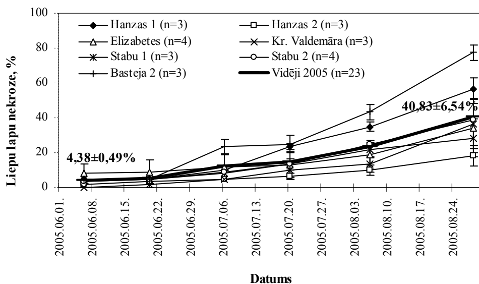
3.3. att. Liepu lapu nekrozes attīstība Rīgas centrā 2005. gada vasarā (vidēji pētījuma vietā 3-5 kokiem ±SE).
