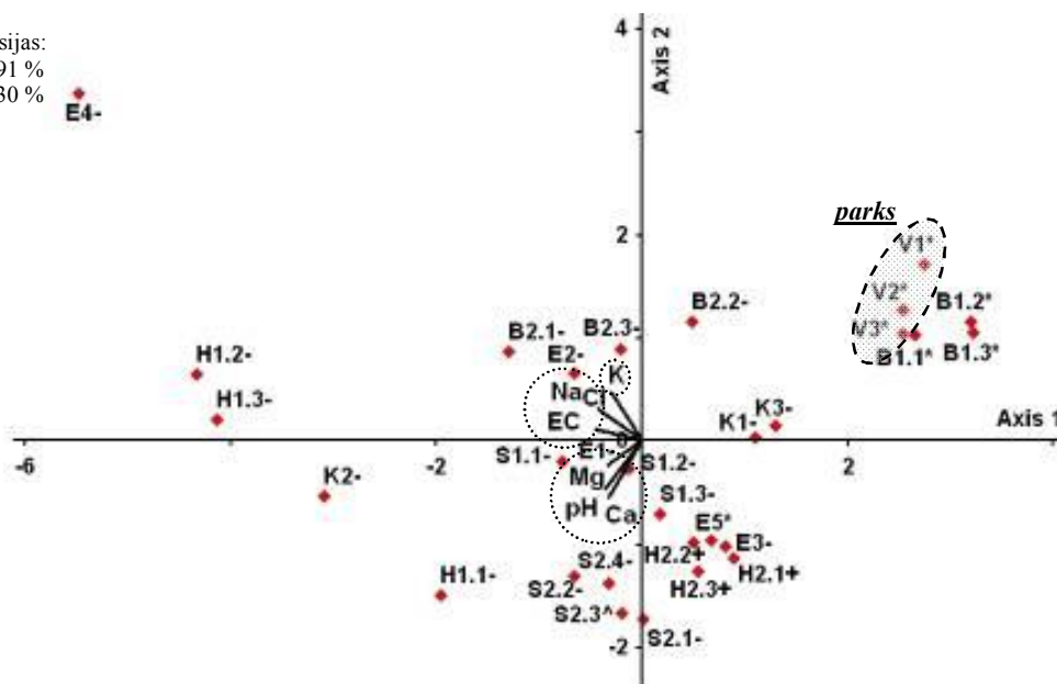
4.5. att. Pētīto parauglaukumu sniega ūdens ķīmiskā sastāva (2004. gada 4. decembra dati) izvietojums ar komponentanalīzi nodalītajās asīs. (* - veselīga; ^ - viegli bojāta; + - vidēji bojāta un - stipri bojāta liepa.)
