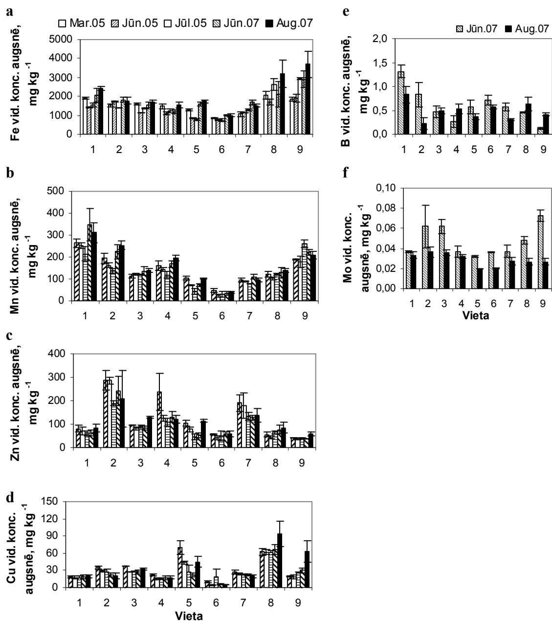
3.17. att. Mikroelementu koncentrācija (mg·kg -1 ) Rīgas ielu apstādījumu augsnē 2005. un 2007. gadā (vidējā koncentrācija 3-5 pētījuma vietas kokiem ±SE).
