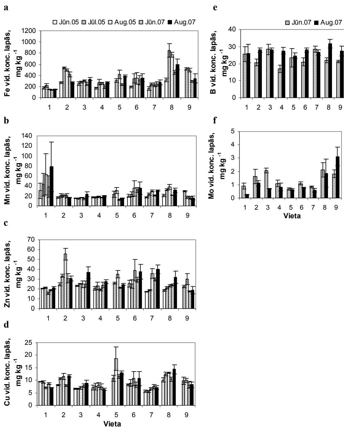
3.21. att. Mikroelementu uzkrāšanās Rīgas ielu apstādījumu liepu lapās 2005. un 2007. gadā (vidējā koncentrācija 3-5 pētījuma vietas kokiem \pm SE).
