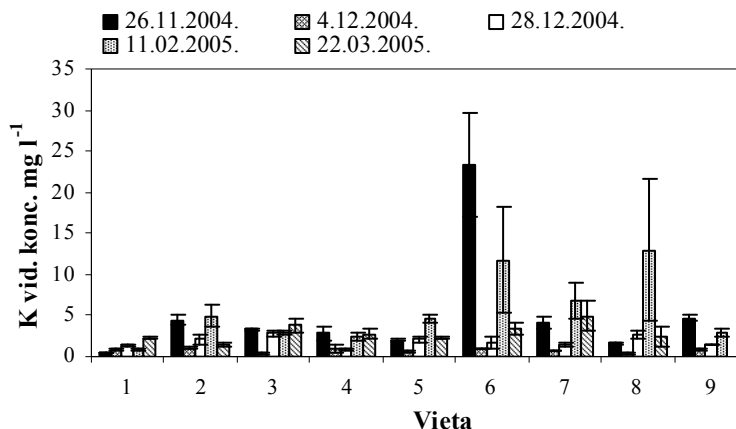
3.11. att. K vidējā koncentrācija (mg·l -1 ) Rīgas centra sniega ūdens paraugos 2004./2005.g. ziemā (vidējā koncentrācija 3–5 pētījuma vietas kokiem ±SE).
