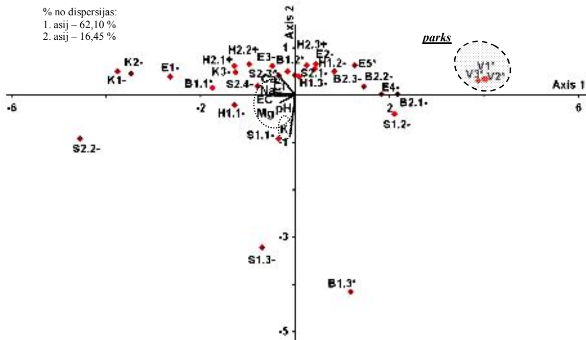
4.7. att. Pētīto parauglaukumu sniega ūdens ķīmiskā sastāva (2005. gada 11. februāra dati) izvietojums ar komponentanalīzi nodalītajās asīs. (* - veselīga; ^ - viegli bojāta; + - vidēji bojāta un – stipri bojāta liepa.)
