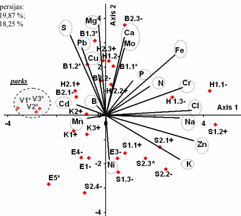
4.17. att. Pētīto parauglaukumu liepu lapu ķīmiskā sastāva (18 elementi, 2007. gada jūnija dati) izvietojums ar komponentanalīzi nodalītājās asīs. (* - veselīga; ^ - viegli bojāta; + - vidēji bojāta un – stipri bojāta liepa).
