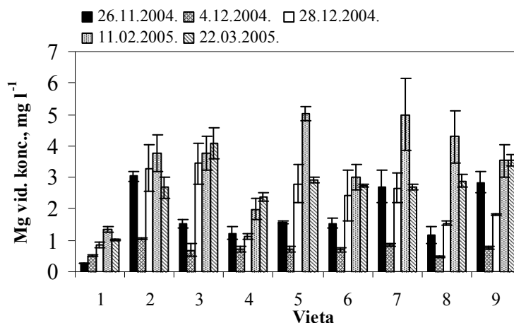
3.13. att. Mg vidējā koncentrācija ( \text{mg}\cdot\text{l}^{-1} ) Rīgas centra sniega ūdens paraugos 2004./2005.g. ziemā (vidējā koncentrācija 3-5 pētījuma vietas kokiem \pm\text{SE} ).
