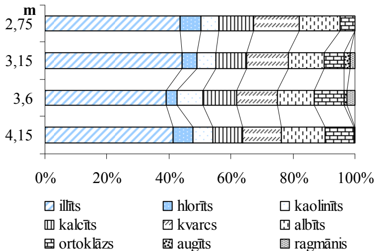
4.6. attēls. Minerālu fāžu kvantitatīvā attiecība glaciģēno ( gQ_3ltv ) (2,75 un 3,15 m) un glaciolimnisko ( glQ_3ltv ) (3,6 un 4,15 m) nogulumu paraugos < 2 \mu m frakcijā no Ulmāles pētījuma iecirkņa
