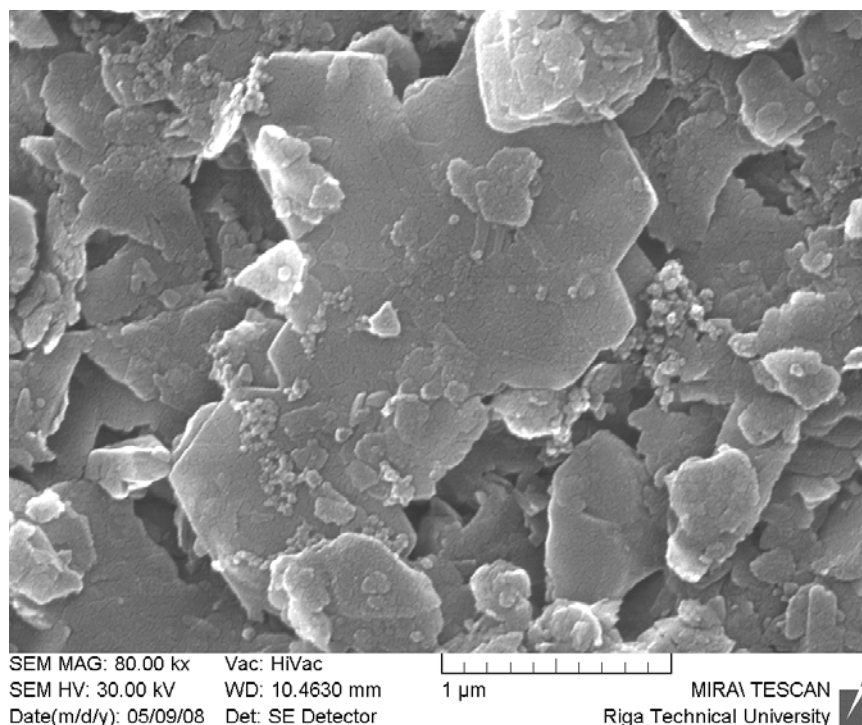
4.12. attēls. Illīta kristalītu koalescences augšana un latiņveida kristalīti uz heksagonālo kristalītu virsmas glaciolimniskas ģenēzes ( glQ_3ltv ) mālaino nogulumu paraugā no Ulmāles pētījuma iecirkņa
