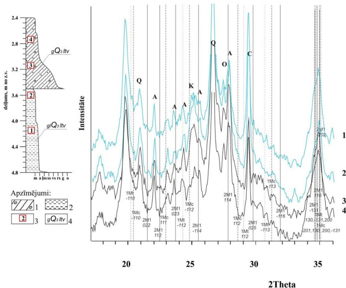
5.6. attēls. XRD spektri 2\theta posmā no 20\text{--}36^\circ paraugiem
