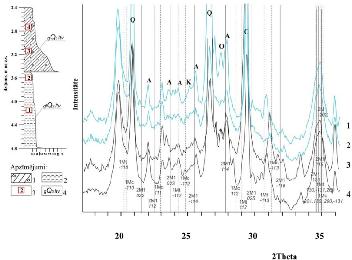
5.8. attēls. XRD spektri 2\theta posmā no 20\text{--}36^\circ paraugiem
