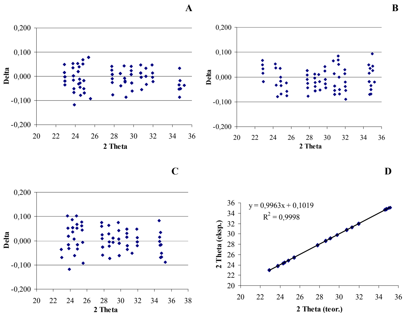
4.2. attēls. Illīta politipu maksimumu nobīde (delta) 2\theta skalā ar teorētiskajiem rezultātiem dažādu frakciju paraugiem no Ulmāles un Kupravas pētījuma iecirkņiem.
