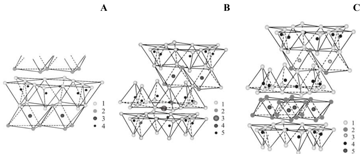
2.1. attēls. Mālu minerālu struktūras. A – shematiska kaolinīta struktūra, pēc Grima (Grim 1962); B – shematiska muskovīta struktūra, kas ir radniecīga illīta struktūrai, pēc Grima (Grim 1962); C – shematiska hlorīta struktūra, pēc Grima (Grim 1962);
