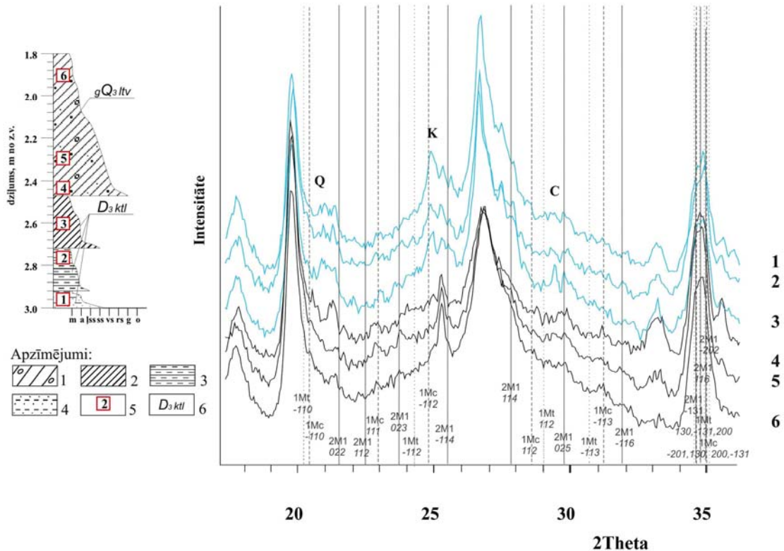
5.7. attēls. XRD spektri 2θ posmā no 20–36° paraugiem
