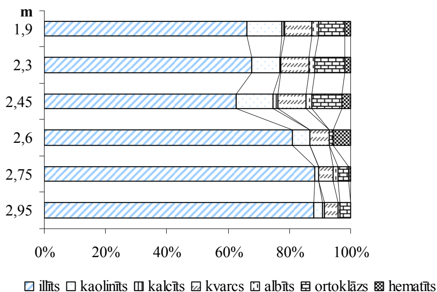
4.7. attēls. Minerālu fāžu kvantitatīvā attiecība glaciģēno nogulumu ( gQ_3ltv ) (1,9–2,45 m) un pamatiežu ( D_3ktl ) (2,6–2,95 m) paraugos < 2 \mu\text{m} frakcijā no Kupravas pētījuma iecirkņa
