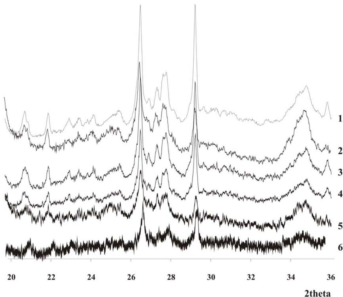
5.2. attēls. Analizējamo paraugu XRD spektri, kuru iegūšanai izmantoti dažādi uzņemšanas parametri
