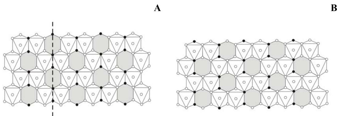
2.2. attēls. Shematiskais trans -vakanto un cis -vakanto pozīciju izkārtojums oktaedru kārtā; A – OH grupas oktaedru kārtā izkārtotas trans -pozīcijās, novērojama simetrijas plakne; B – OH grupas oktaedru kārtā izkārtotas cis -pozīcijās, simetrijas plakne nav novērojama, pēc Meinerā (Meunier 2005)
