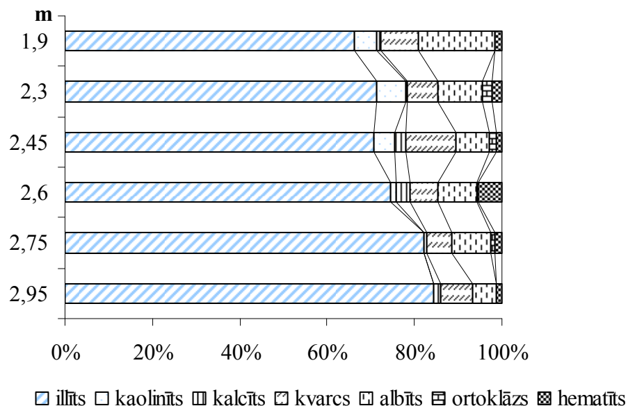
4.9. attēls. Minerālu fāžu kvantitatīvā attiecība glaciģēno nogulumu ( gQ_3/tv ) (1,9–2,45 m) un pamatiežu ( D_3/ktl ) (2,6–2,95 m) paraugos < 1 \mu m frakcijā no Kupravas pētījuma iecirkņa
