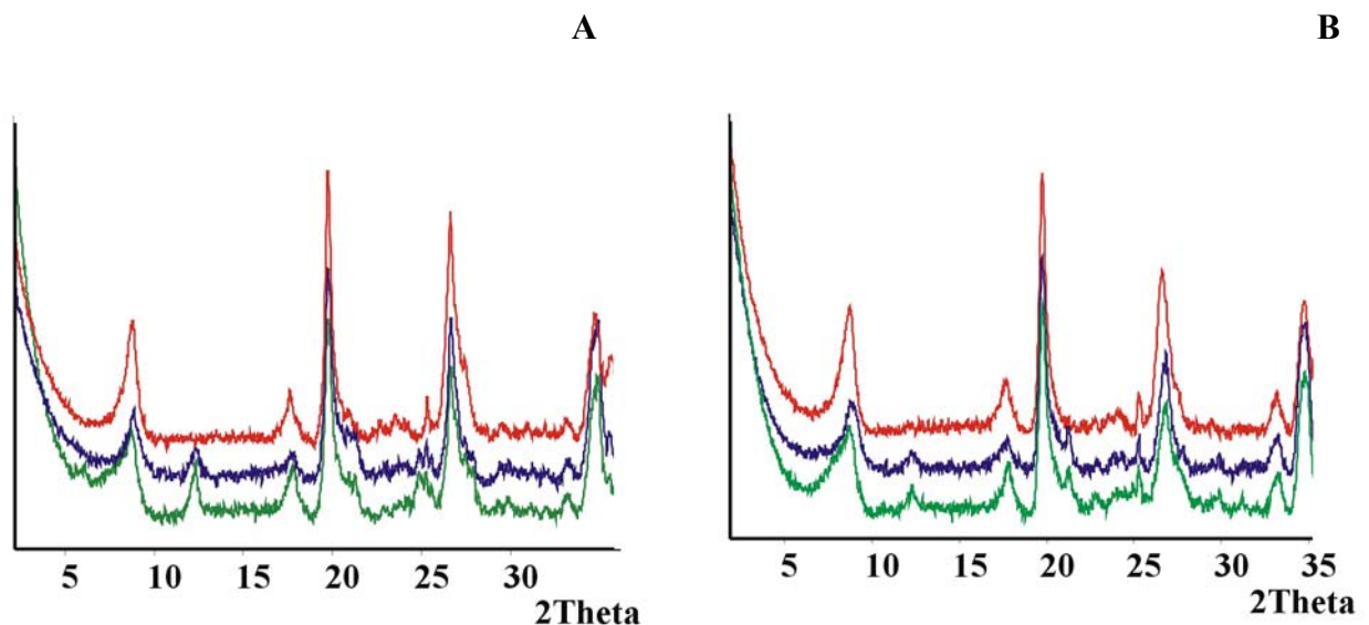
4.4. attēls. Neteksturēto dažādi apstrādāto paraugu XRD spektru piemēri no Kupravas pētījuma iecirkņa: A – glaciģēno nogulumu ( gQ_3ltv ) paraugu spektri; B – zem glaciģēnajiem nogulumiem ieguļošo mālaino pamatiežu ( D_3ktl ) paraugu spektri Apzīmējumi: — paraugs apstrādāts karsējot 2 h pie 550^\circ C ; — paraugs apstrādāts ar etilēnglikolu 12 h pie 70^\circ C ; — neapstrādāts nogulumu paraugs
