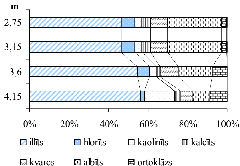
4.8. attēls. Minerālu fāžu kvantitatīvā attiecība glacigēno ( gQ_3ltv ) (2,75 un 3,15 m) un glaciolimnisko ( glQ_3ltv ) (3,6 un 4,15 m) nogulumu paraugos < 1 \mu m frakcijā no Ulmāles pētījuma iecirkņa
