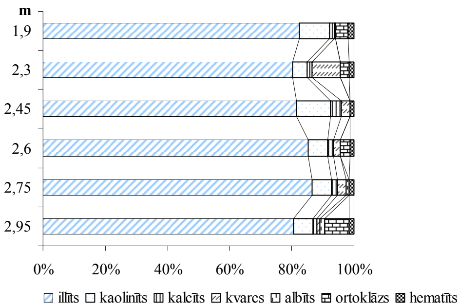
4.11. attēls. Minerālu fāžu kvantitatīvā attiecība glaciģēno nogulumu ( gQ_3ltv ) (1,9–2,45 m) un pamatiežu ( D_3ktl ) (2,6–2,95 m) paraugos < 0,4 \mu m frakcijā no Kupravas pētījuma iecirkņa
