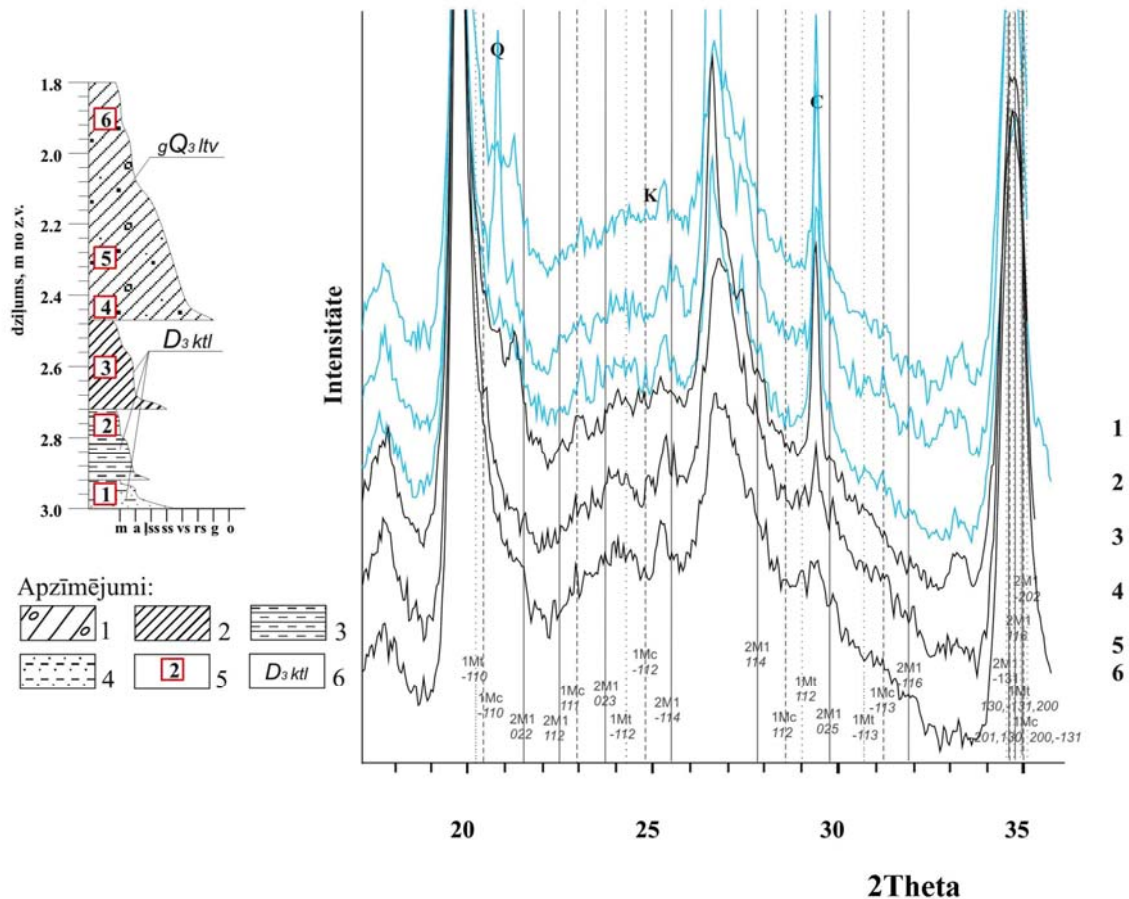
5.9. attēls. XRD spektri 2\theta posmā no 20–36° paraugiem < 0,4 μm un ģeoloģiskais griezumā no Kupravas pētījuma iecirkņa Apzīmējumi: ģeoloģiskais griezumā – 1 – smilšmāla morēna; 2 – smilšmāls; 3 – aleirītiski māli; 4 – aleirītiska smalka smiltis; 5 – parauga numurs; 6 – nogulumu ģenēze un ģeoloģiskais vecums; m – māli; a – aleirīti; ļss – ļoti smalka smiltis; ss – smalka smiltis; vs – vidēji smalka smiltis; rs – rupja smiltis; g – grants; o – oļi; XRD spektri – 1; 2 un 3 – zem glacigēnajiem nogulumiem iegulošo nogulumu ( D_3ktl ) XRD spektri; 4; 5 un 6 – glacigēno nogulumu ( gQ_3ltv ) XRD spektri. Illīta polītipiem raksturīgo nebazālo maksimumu atrašanās vieta: 2M_l – melna līnija; 1Mc_v – pārtraukta līnija; 1Mtv – punktēta līnija; Q – kvarcs; K – kaolīnīts; A – albīts; C – kalcīts; H – hematīts
