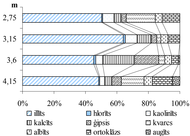
4.10. attēls. Minerālu fāžu kvantitatīvā attiecība glaciģēno ( gQ_3ltv ) (2,75 un 3,15 m) un glaciolimnisko ( glQ_3ltv ) (3,6 un 4,15 m) nogulumu paraugos < 0,4 \mu m frakcijā no Ulmāles pētījuma iecirkņa
