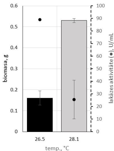
2. attēls. L. edodes 3565 micēlija biomasas (g/100mL) un lakāzes aktivitāte (●, U/mL) iesala ekstrakta (½ MEB) barotnēs (140rpm) pie dažādām inkubācijas temperatūrām. Apzīmējumi: “***” p-vērtība < 0.01
