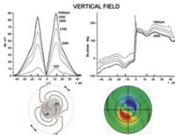
Magnētiskā lauka aina (lejā pa kreisi), ko zīmējusi datorprogramma no eksperimentā iegūtiem mērījumiem (augšā) principā sakrīt ar teorētiski aprēķināto (lejā pa labi)
