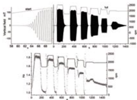
Eksperimenta laikā mērīerīču nolasīto datu grafiskais pieraksts (magnētiskā lauka amplitūdas (eksperimenta 58. līdz 70. sekunde un visā eksperimenta gaitā) augšā un frekvences grafiki lejā)
