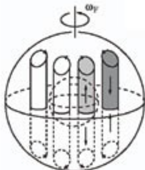
Cikloni un anticikloni, kuri atmosfērā ir gandrīz plakani gar pašu Zemes virsu, Zemes kodola iegūst garu cilindru formu
