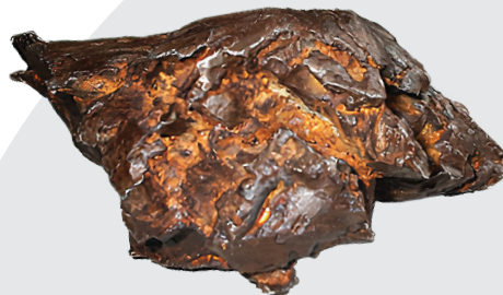
Sihotealina meteorīts – dzelzs oktaedrīts. Paraugs no LU Muzeja F. Candra un Latvijas astronomijas kolekcijas. 1947. gadā nolija meteorītu lietus ar kopīgo masu ap 70 t, izveidojot 24 trieciena krāterus
