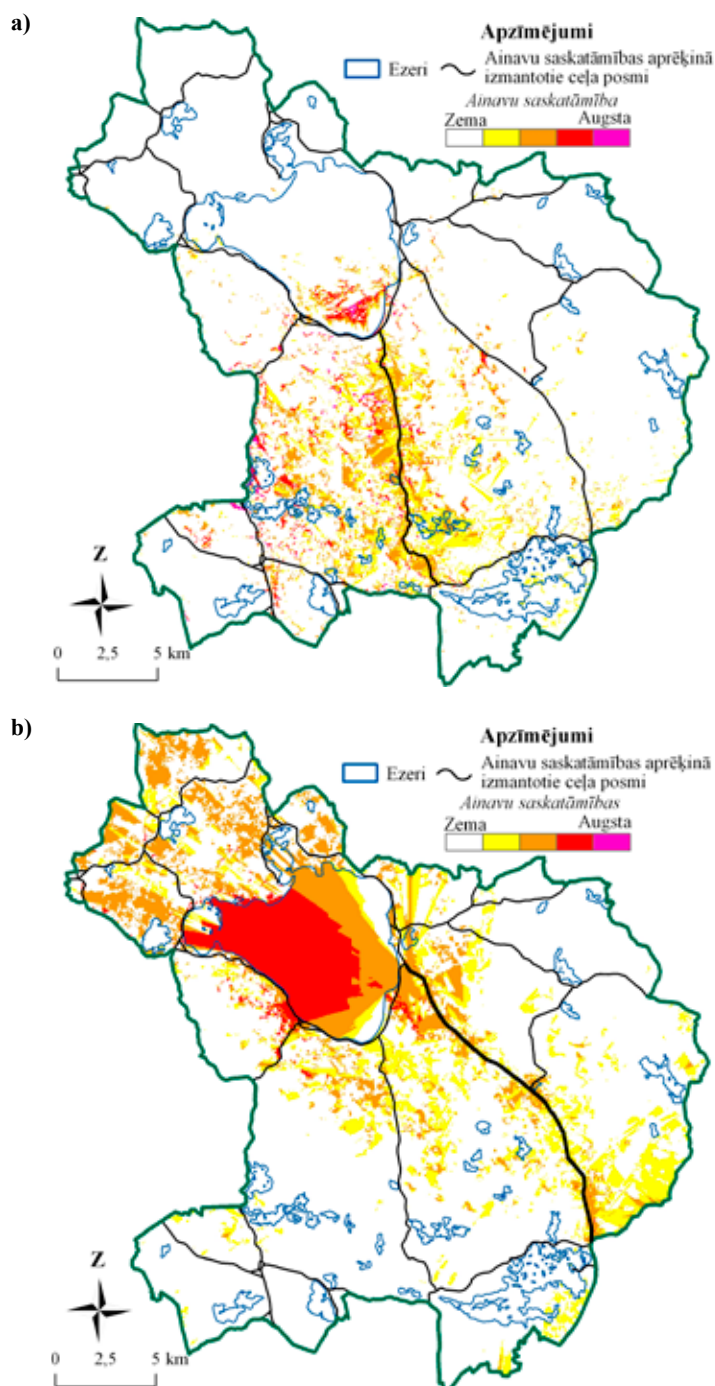
3.26. attēls. Saskatāmības modeļēšanas rezultāti atsevišķiem ceļu posmiem
