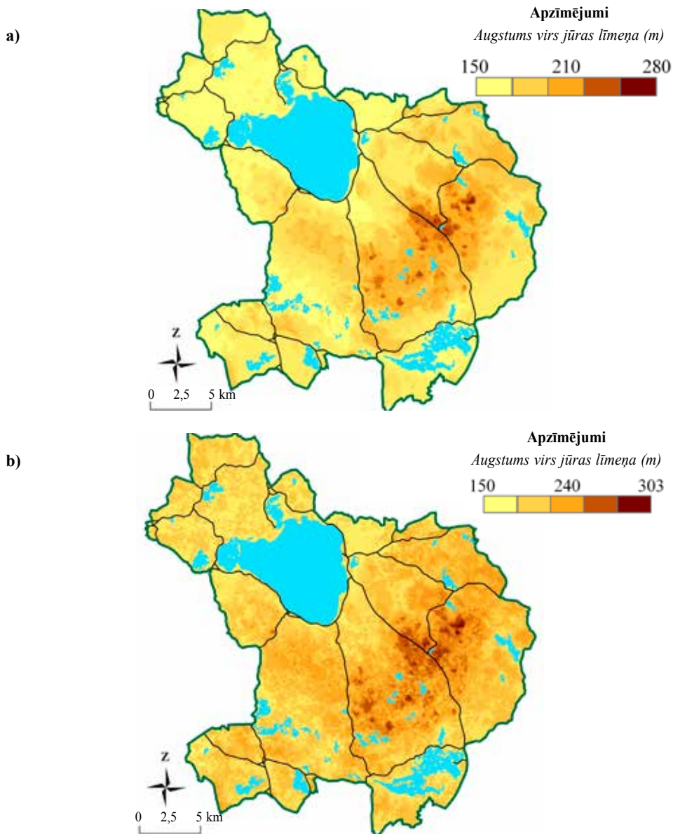
3.23. attēls. Rāznas nacionālā parka reljefa modelis (a) un zemsedzes virsmas augstuma modelis, kurā apvienots reljefs ar apauguma tipa augstumu (b)
