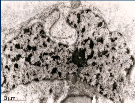
Kodola novecošana augu lapu šūnā (Philips 300)
