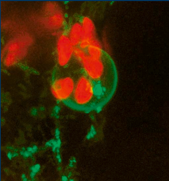
3D attēls konfokālajā lāzerskenējošajā mikroskopā. Kodola un hloroplastu novietojums šūnā. Kodola diametrs – 20 mikrometri (Leica DM RA-2)
