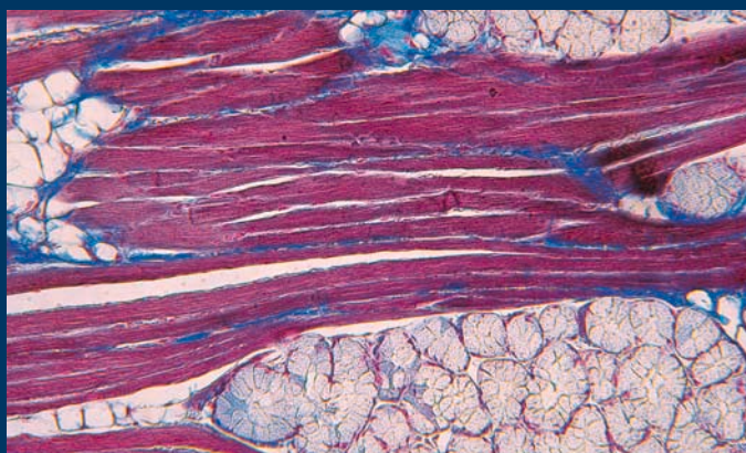
Cilvēka audi (Leica DM 2000)
